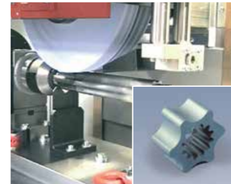
Außenprofil von Pumpenrotoren
