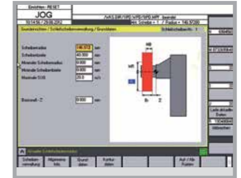
Schleifscheibenparameter
