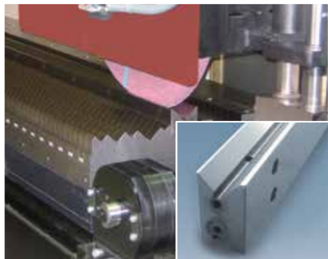
Führungsleiste
