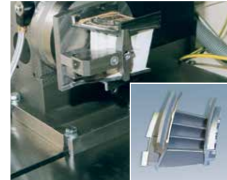
Turbinenleit- und -laufschaufel
