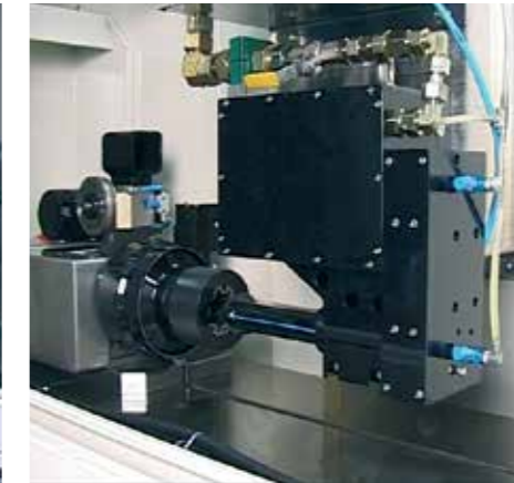
Horizontal-Innenschleifeinrichtung , Schleifscheiben \varnothing 25 \dots 70 mm; bis 45.000 \text{ min}^{-1}
