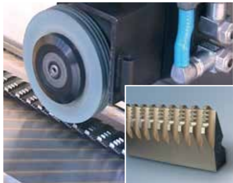
Räumwerkzeug
