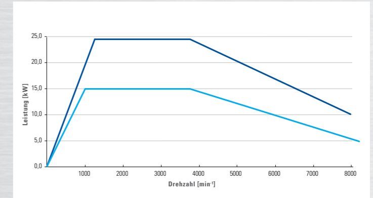
Der Schleifspindeltrieb leistet 15 kW. Optional ist der Antrieb mit 24,5 kW erhältlich
