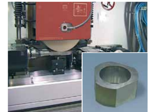
Laufring für Einspritzpumpe
